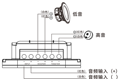
分频器
